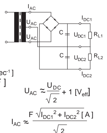
Abb. 8 Gleichrichtung
