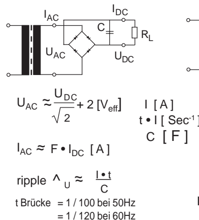
Abb. 7 Gleichrichtung
