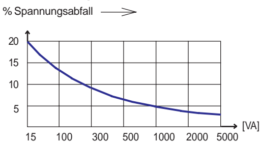
Abb. 2 Spannungsabfall
